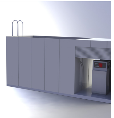
Модель КАЗС 02: 2 вида топлива, 2 колонки, 2 пистолета
