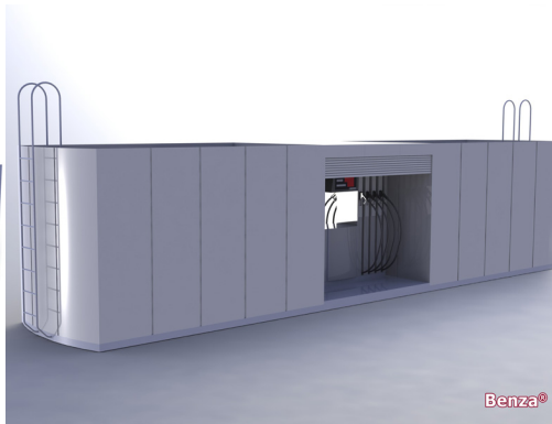
Модель КАЗС 03: 4 вида топлива, 2 колонки, 8 пистолетов
